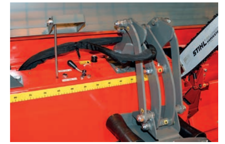
AC 10 automaattinen ketjunkturin pitää teräketjun aina optimaalisella kireydellä. Ketjun voi vaihtaa kätevästi löysäämällä teräketjun kuvan vipua kääntämällä - ilman työkaluja!
