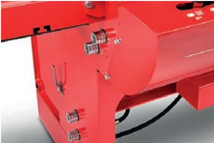
Des flexibles hydrauliques peuvent être facilement raccordés à la machine grâce à des raccords rapides en accessoire.
