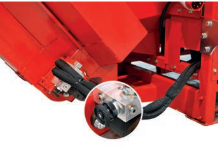
Poistokuljettimen nopeudensäätöventtiili helposti asennettavana lisävarusteena.
