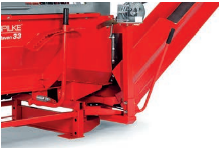
Vakiona hydraulivetoinen, kääntyvä poistokuljetin.
