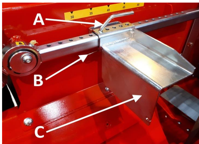
Abb. 14: Position des Messgeräts für kleine Holz unter 25 cm
