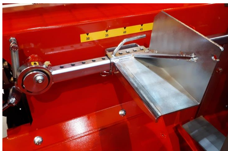
Abb. 15: Position des Messgeräts für großes Holz mit einem Durchmesser über 25 cm.
