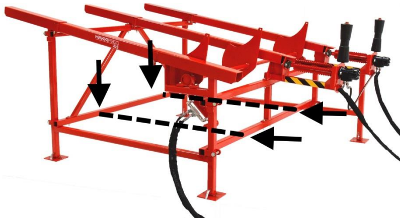
Kuva 1. Koneen nostokohdat
