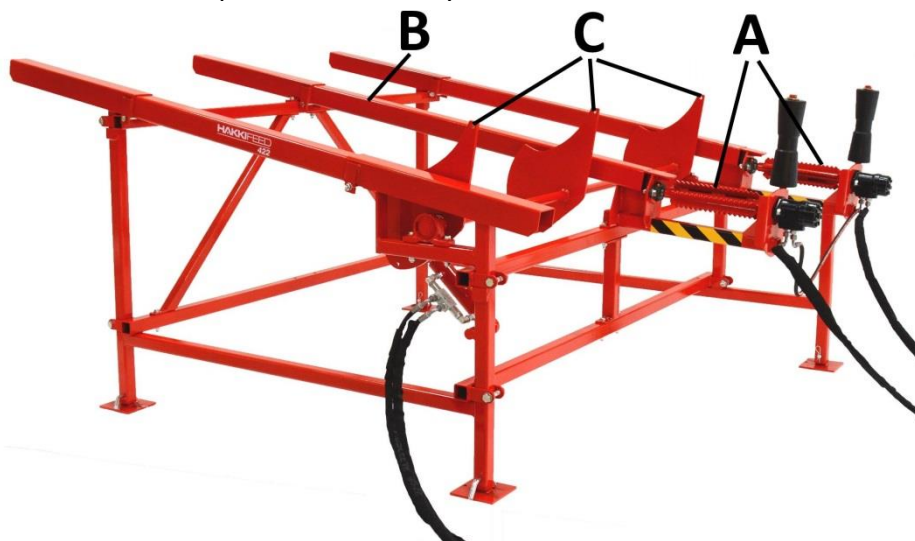
Kuva 2. Koneen pääosat
