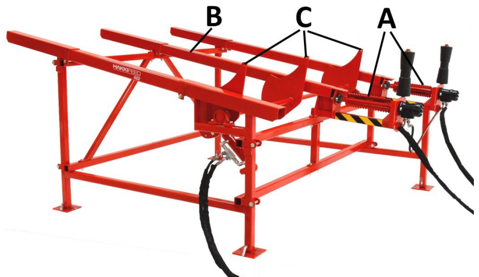
Bild 2. Maskinens huvuddelar
