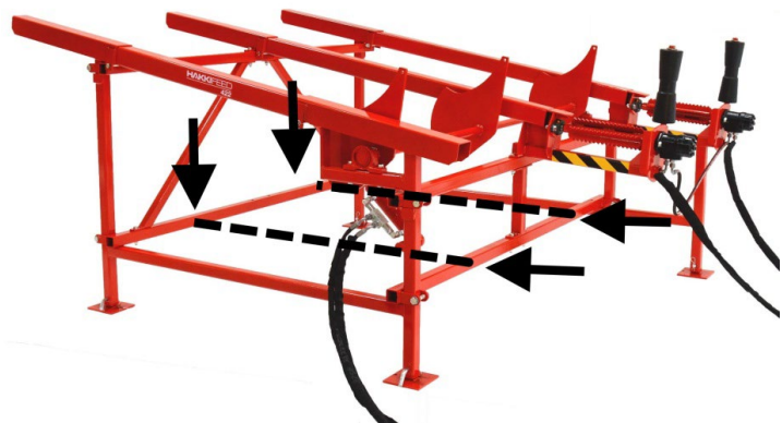
Bild 1. Maskinens lyftpunkter
